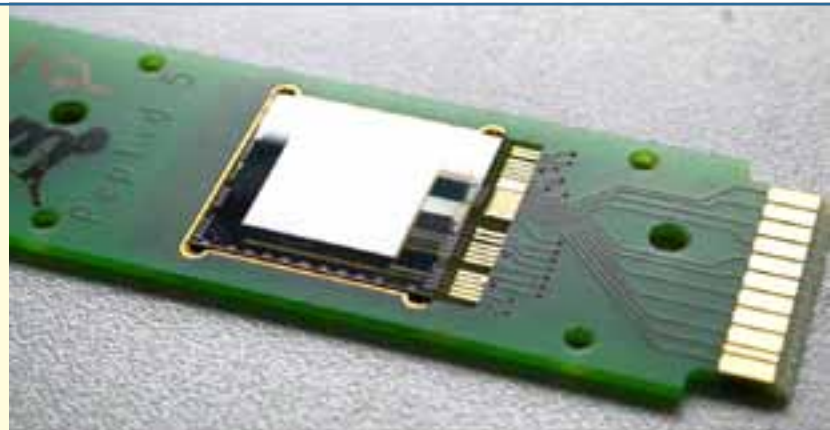
Peptidchip 5 auf seinem PCB-Träger von der Größe eines normalen Objektträgers (75.8 mm x 25.9 mm x 1.0 mm).
