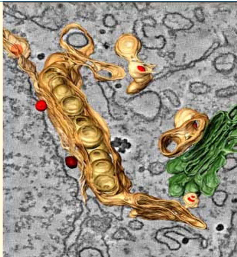
3D-Modell der Kompartimente, in denen Flaviviren replizieren und assembliert werden.
