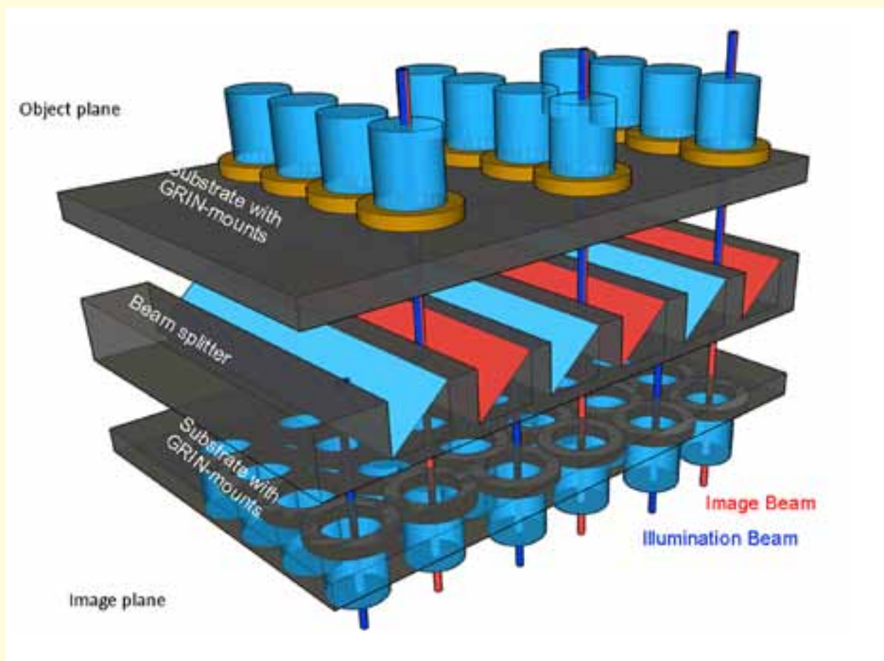
Schematische Darstellung einer miniaturisierten Anordnung von 12 parallel arbeitenden Mikroskopen, realisiert in Schichttechnik mit Gradientenindex-Linsen.
